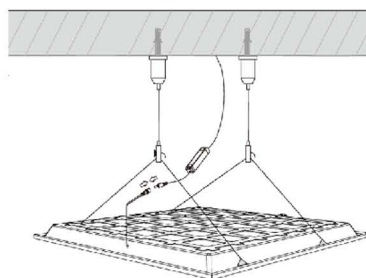
Pendant Type
